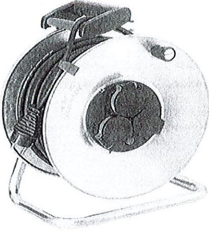
3.34 - 3 x 2,5 mm 30 mt kablolu seyyar makaralı uzatma kablosu
