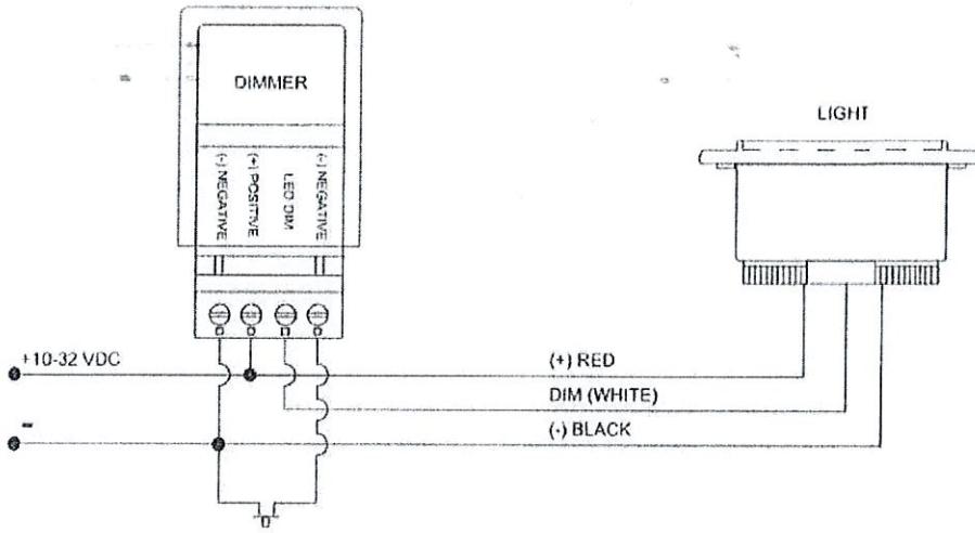
3.41 - 24 v dc 55 w halojen seramik gövdeli lamba
